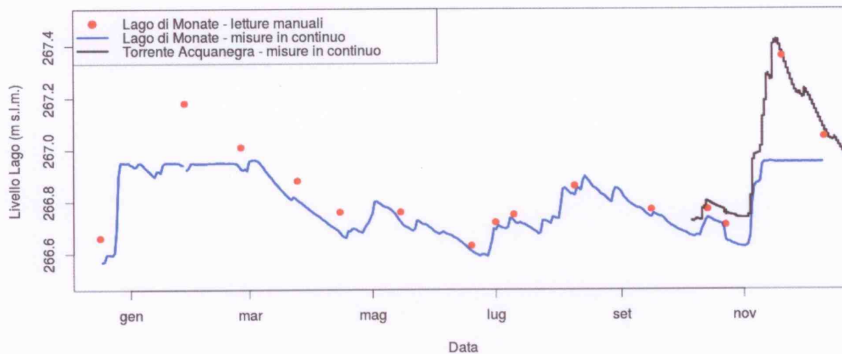
Figura 1. Serie temporali della quota del pelo libero del Lago di Monate (presso idrometro, linea blu) e dell'incile del T. Acquanegra (sezione di misura delle portate, linea nera), oltre alle letture manuali del livello del Lago di Monate (punti rossi).
