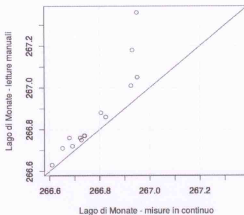
Figura 3. Diagramma di dispersione per il confronto tra le misure manuali e quelle in continuo del livello del Lago di Monate
